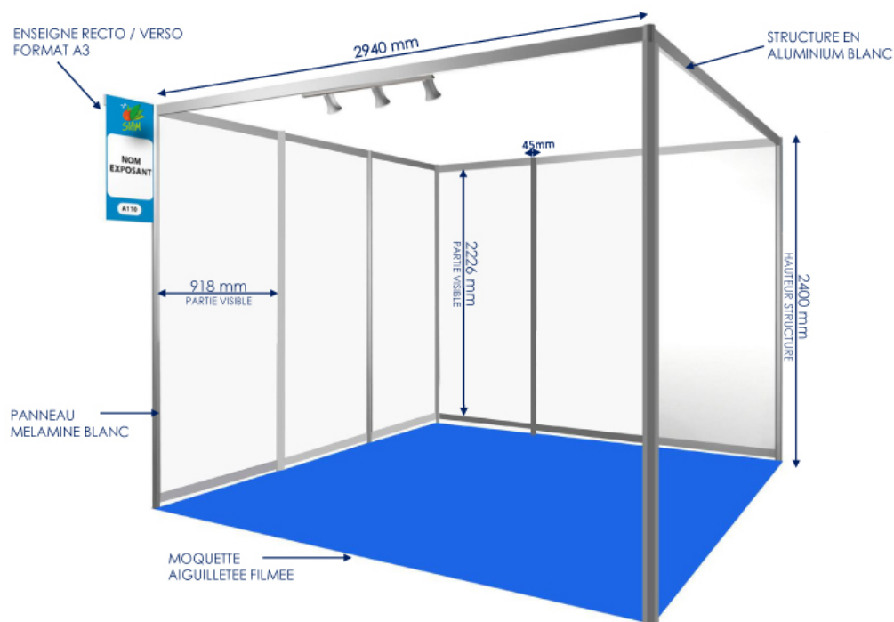
DETAIL STAND MODULAIRE MODELE TYPE : 9M 2 COTES: 3MX3M
